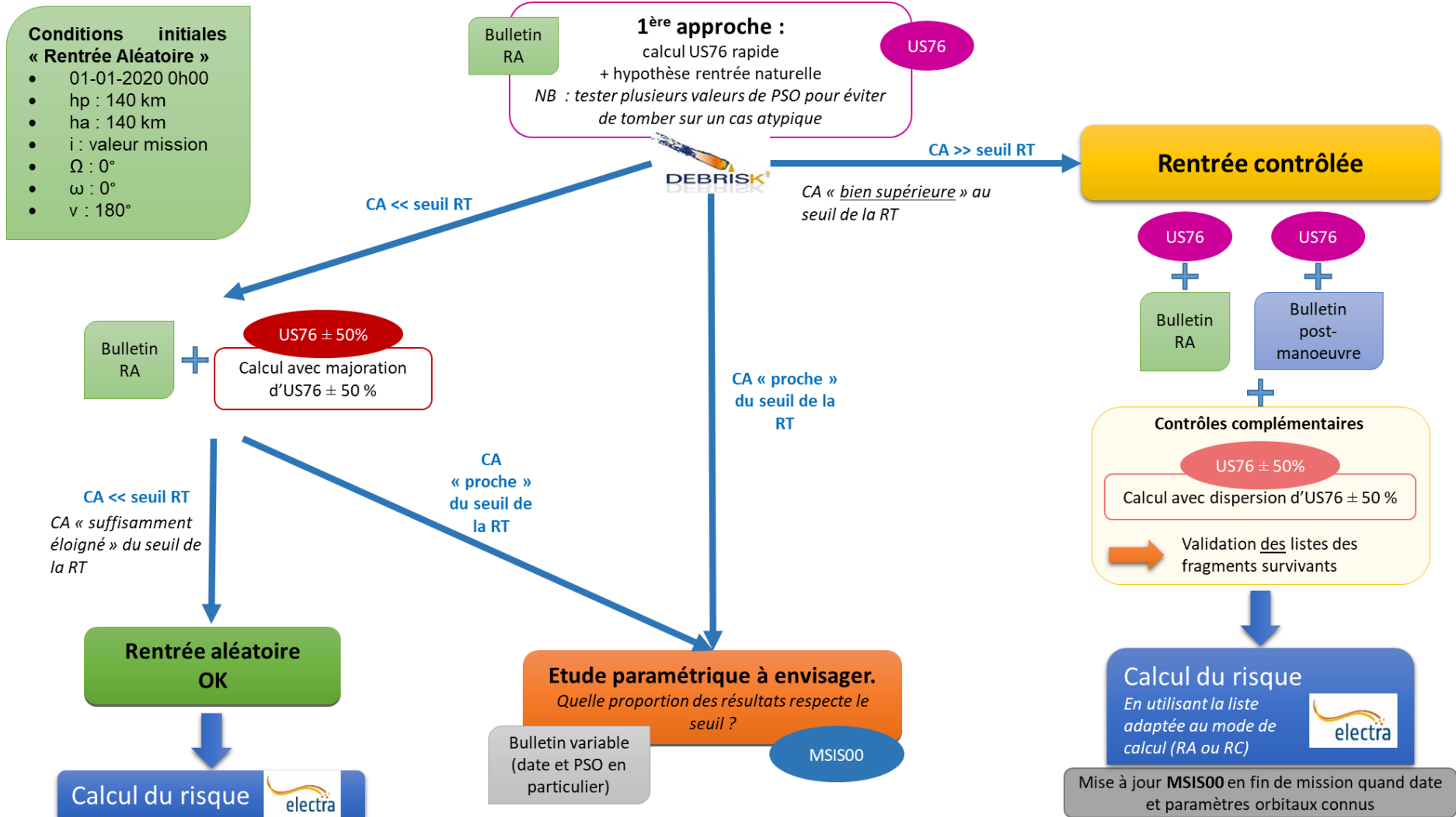
Figure 2 – Schéma des préconisations sur le choix du modèle d’atmosphère et des conditions orbitales
